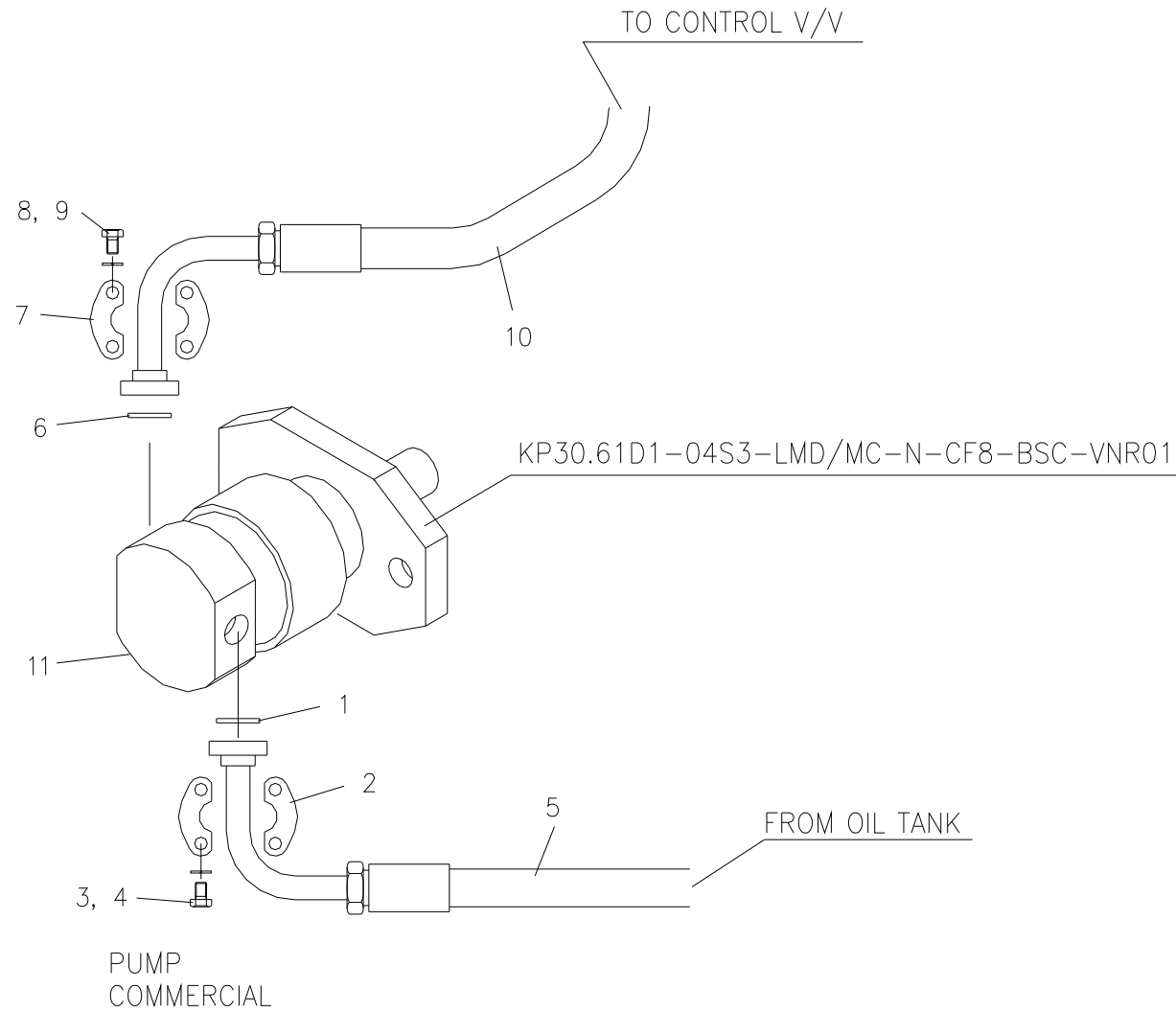
장착 배관 파트 Fig. 8 SCS747L M/T PIPING PART
