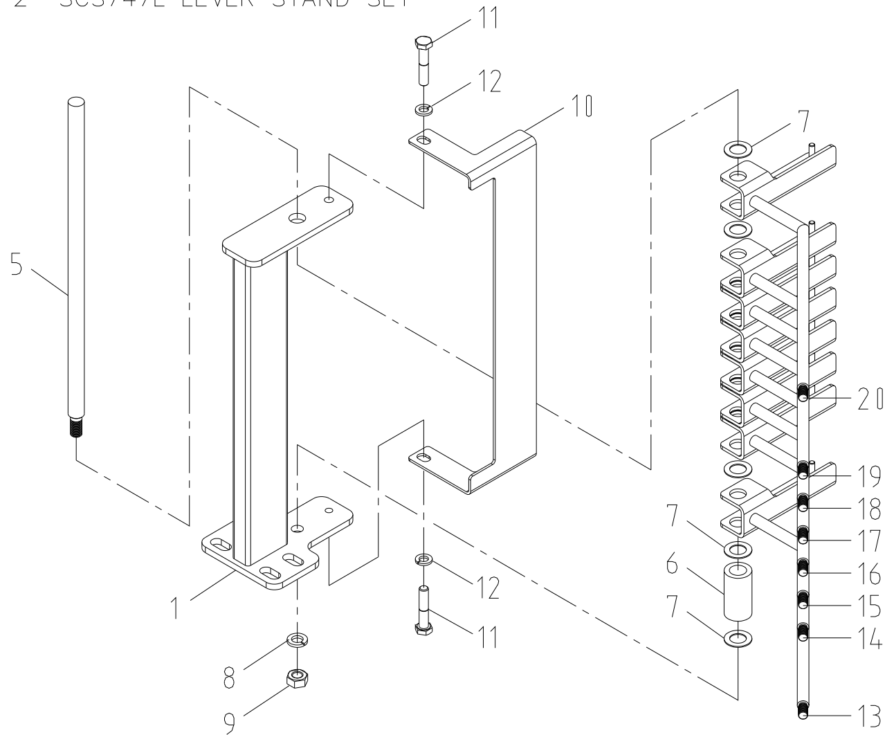
레버 스탠드 셋 Fig. 3-4-2 SCS747L LEVER STAND SET
