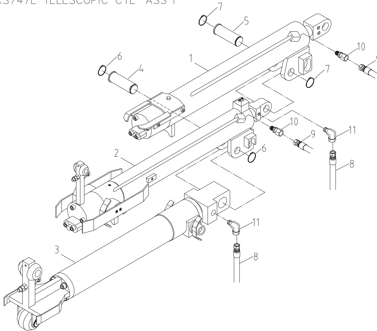
텔레스코픽 실린더 조립체 Fig. 1-1 SCS747L TELESCOPIC CYL' ASS'Y
