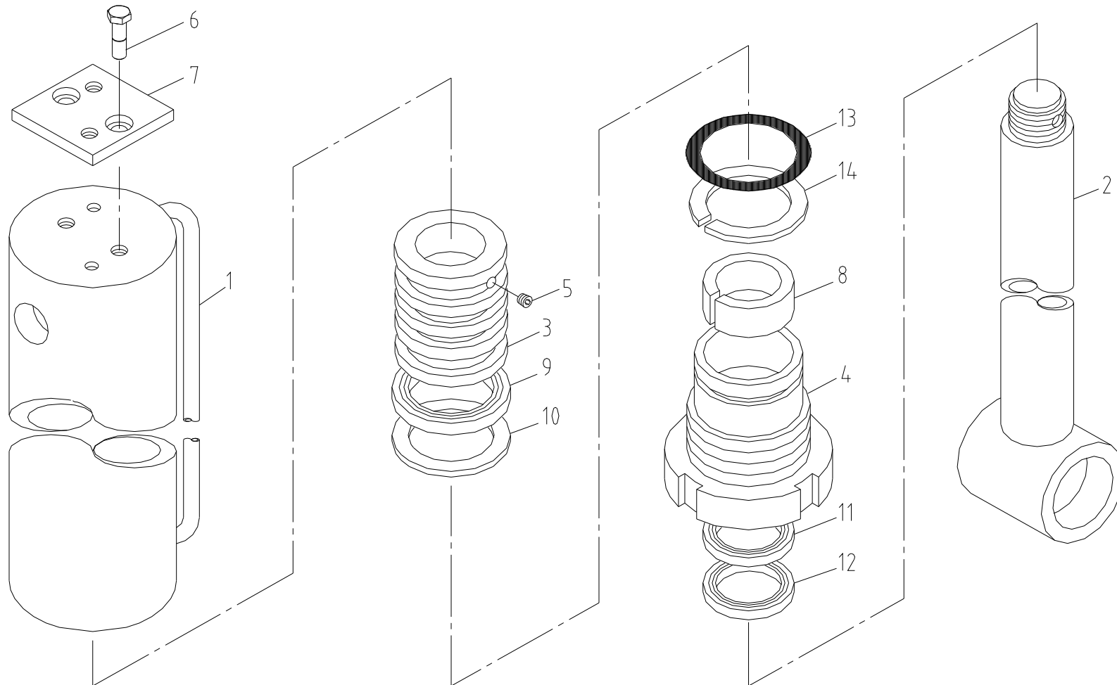
잭 실린더 조립체 Fig. 4-1 SCS746L JACK CYL' ASS'Y
