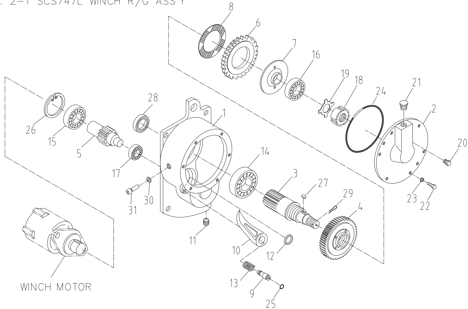
원치 감속기 조립체 Fig. 2-1 SCS747L WINCH R/G ASS'Y
