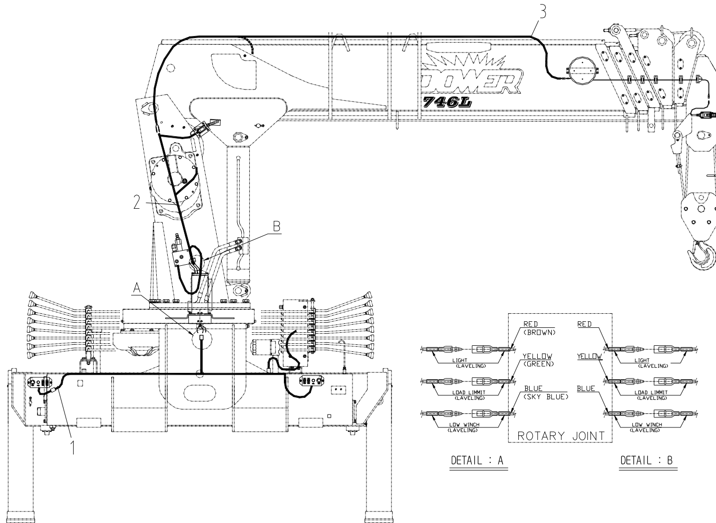
전선 조립체 Fig. 11 SCS747L WIRING ASS'Y
