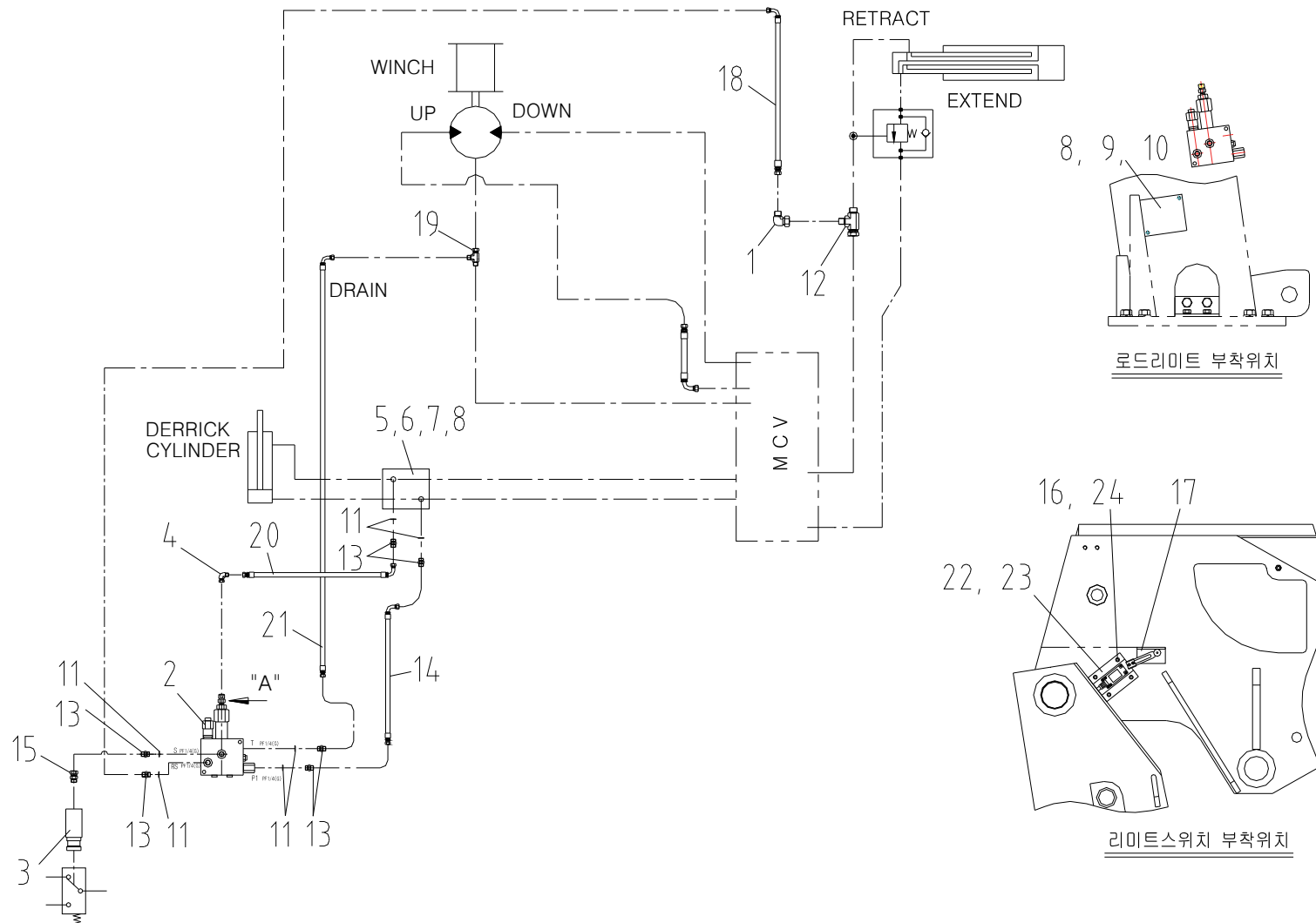
과하중 방지 배관 조립체 Fig. 10 SCS747L OVERWINDING ALARM PIPING ASS'Y
