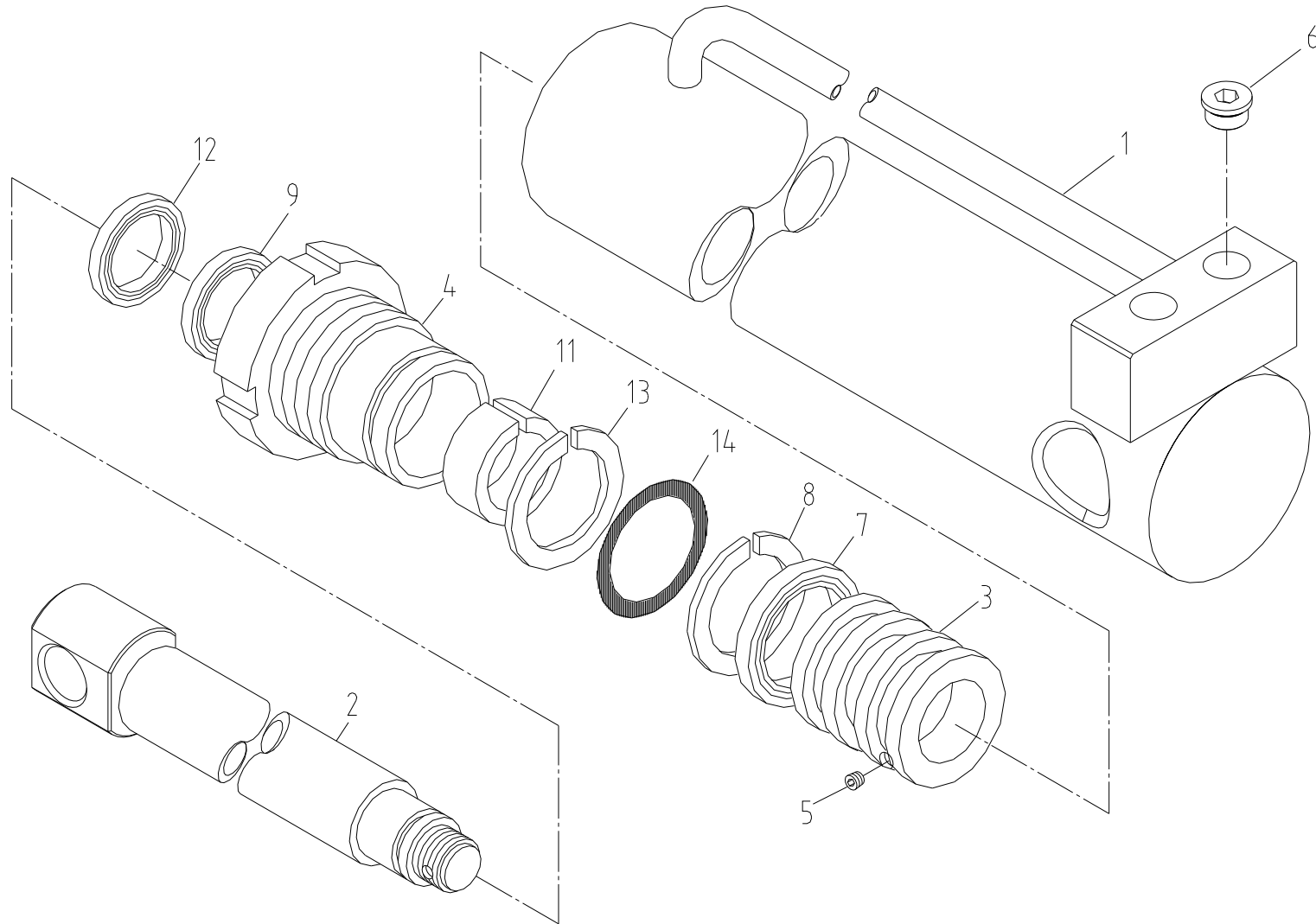
익스펜딩 실린더 조립체 Fig. 4-2 SCS747L EXPANDING CYL' ASS'Y
