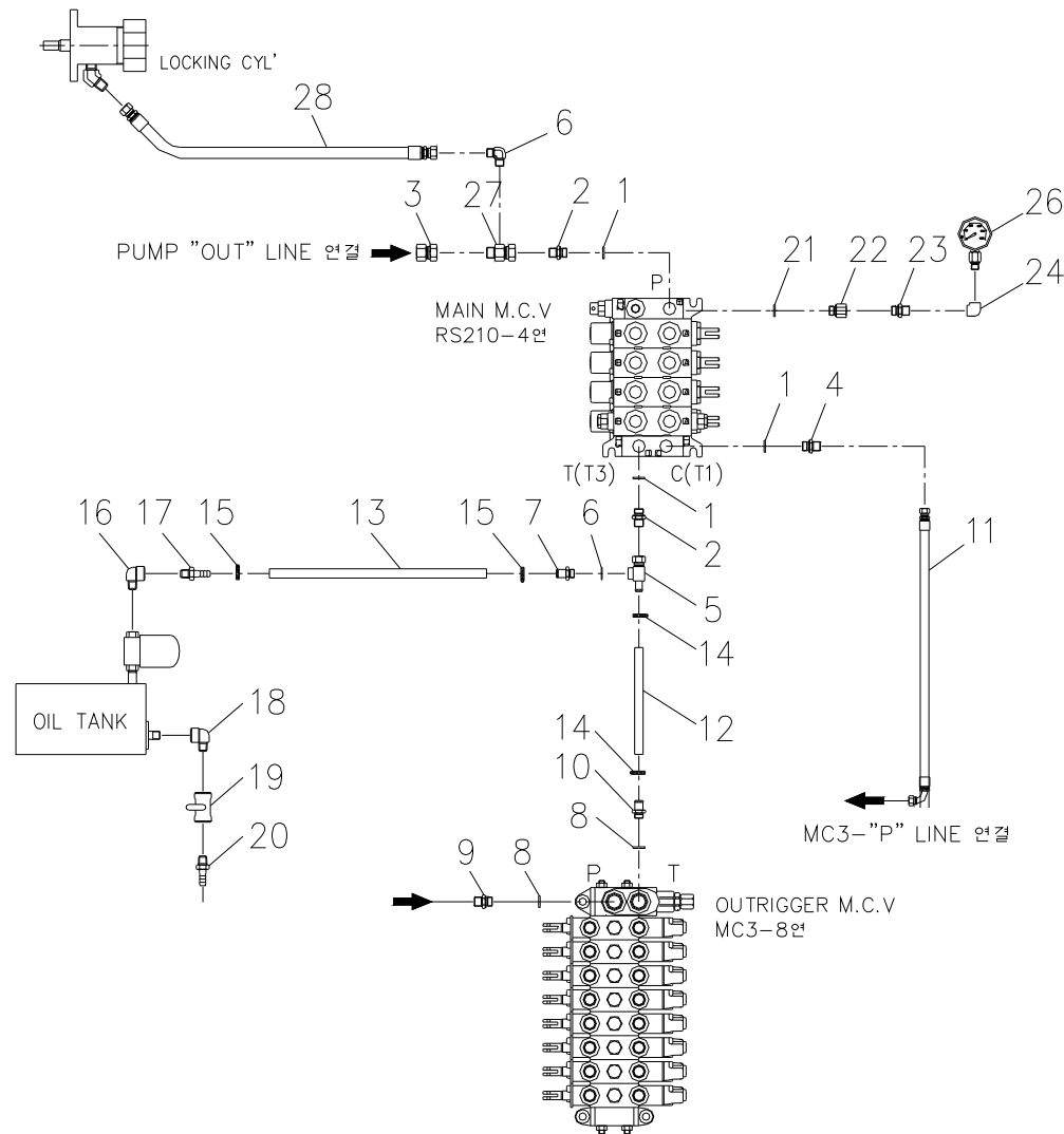
디스트리뷰터 배관 Fig. 5-1 SCS747L DISTRIBUTOR PIPING
