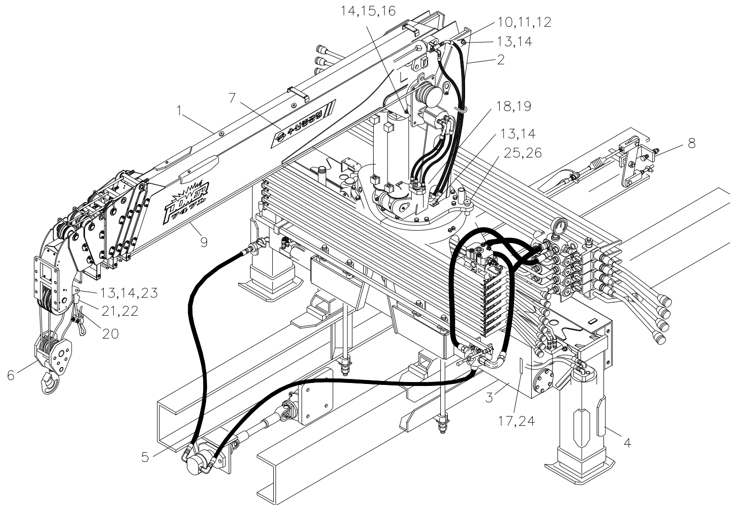
크레인 조립체 (표준형) Fig. 0 SCS747L CRANE ASS'Y (STD)
