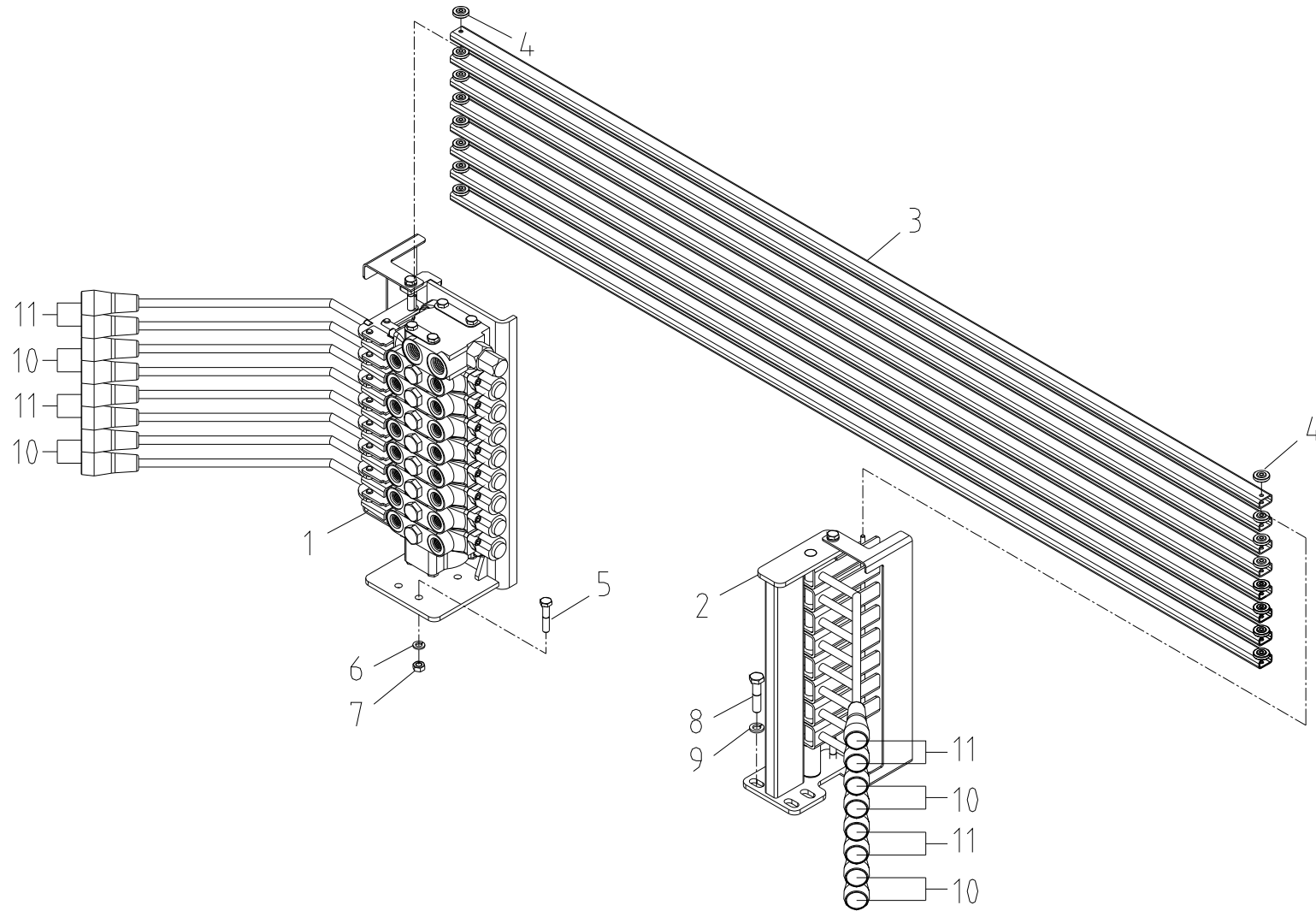
오퍼레이션 아우트리거 조립체 Fig. 3-4 SCS747L OPERATION OUTRIGGER ASS'Y
