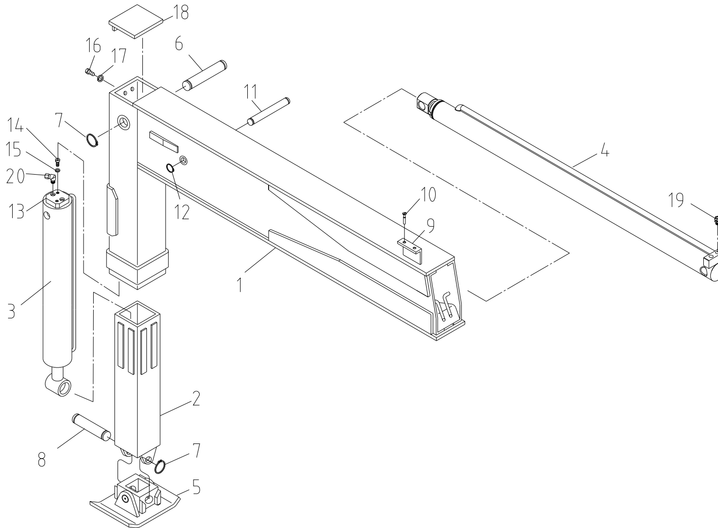
아우트리거 조립체 (8톤) Fig. 4 SCS747L OUTRIGGER ASS'Y(8TON)
